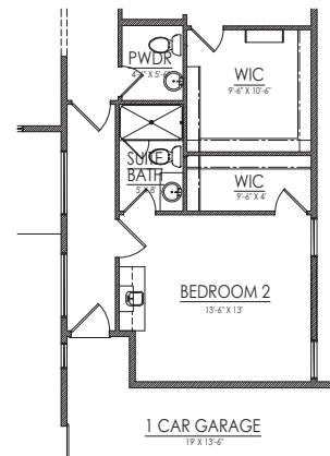
OPTIONAL GRAND SUITE
