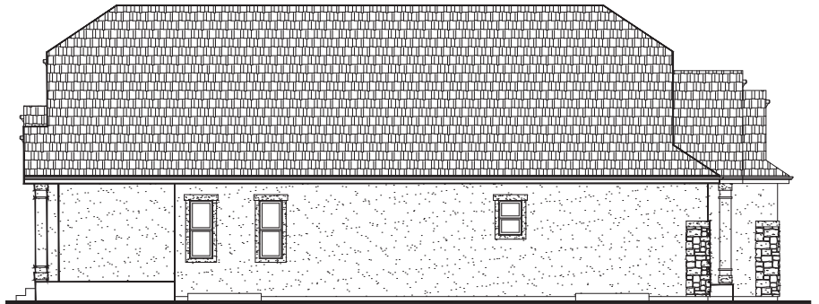
LEFT ELEVATION 'L'
